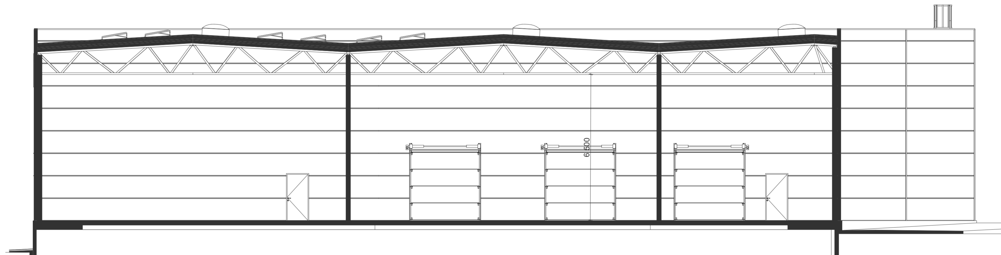
HOONE LÕIGE 2-2 | 1:100
